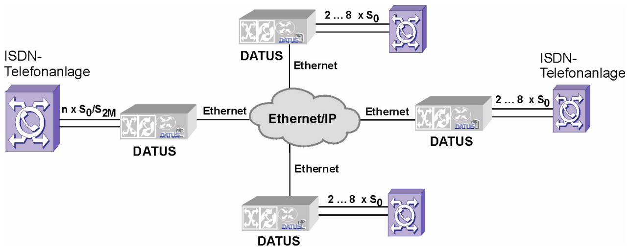
Abb. 1: Anbindung abgesetzter Telefonanlagen über Ethernet-basierte Netze
